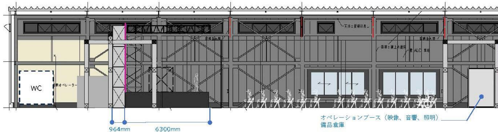
断面図
